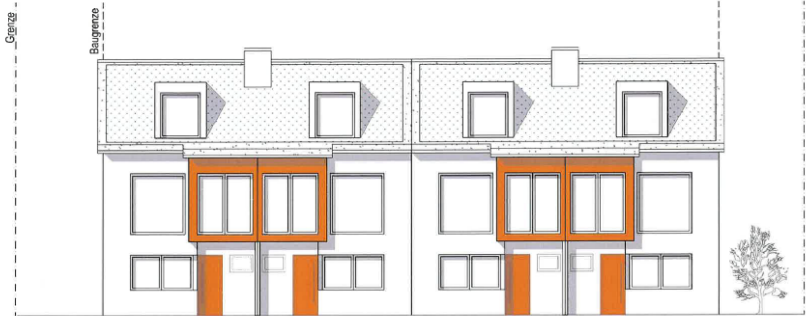
ANSICHT NORD
